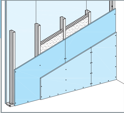
دیوار جداکننده W112
